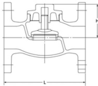
F-F dimension : JIS B 2011 End flanges : JIS B 2239 10K
